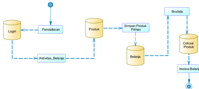
Gambar 1. Komponen Umum Basis Data De Janggelan
